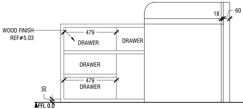
ELEVATION B
