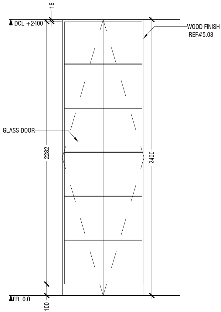
ELEVATION A
